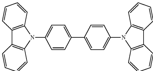
[BCP]
